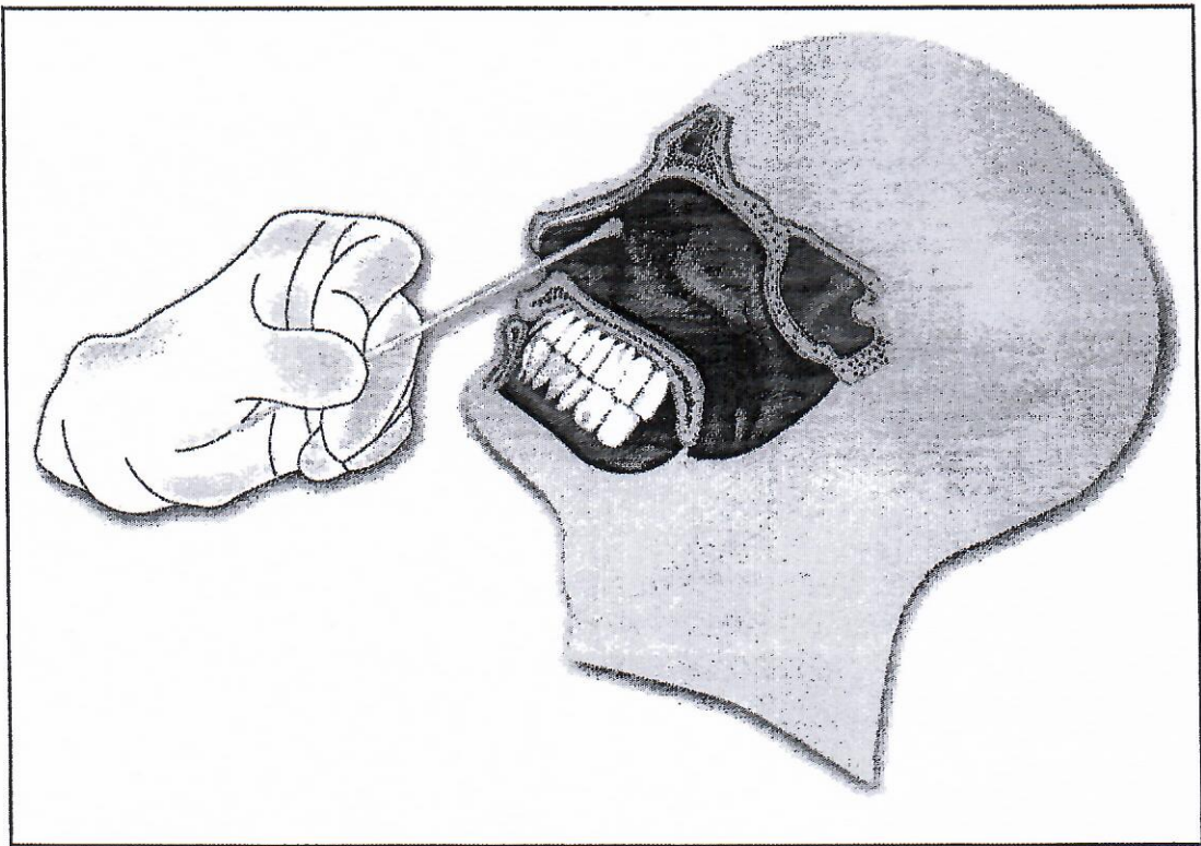
FIGURA 2. Tampone nasale
